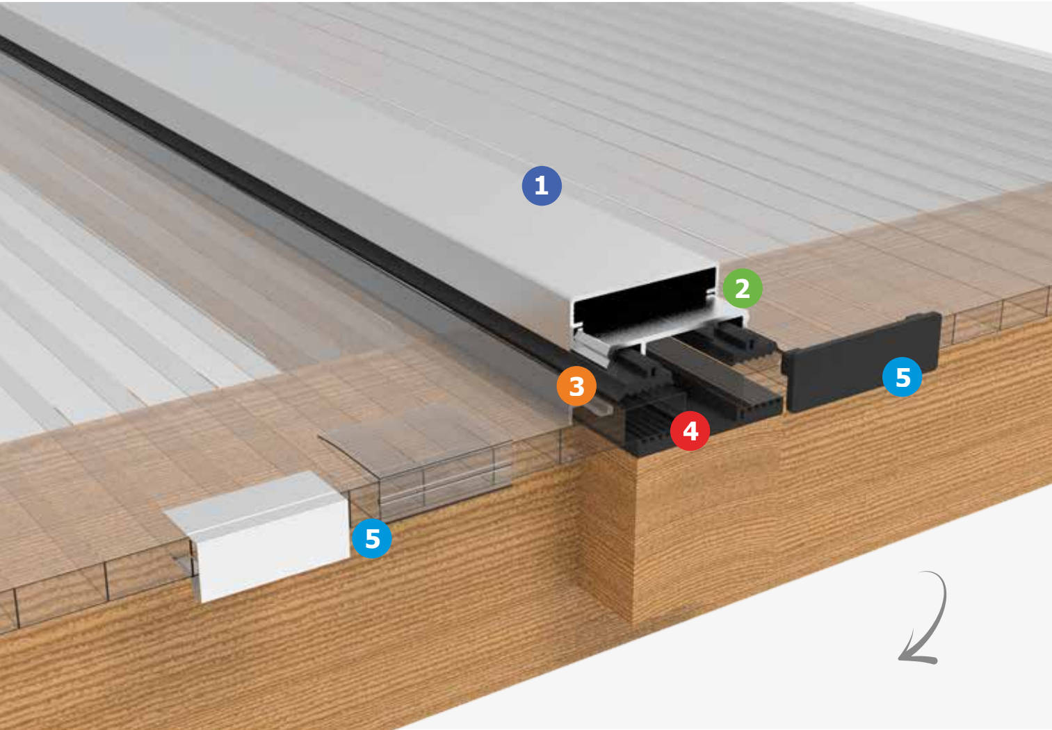
1. ALU-KLIPSCHECKSCHIENE | 2. ALU-FLACHCHECKSCHIENE | 3. DICHTUNGSGUMMI | 4. AUFLEGEKLEB | 5. XXXXXXXXXXXXXXXXXXXX
