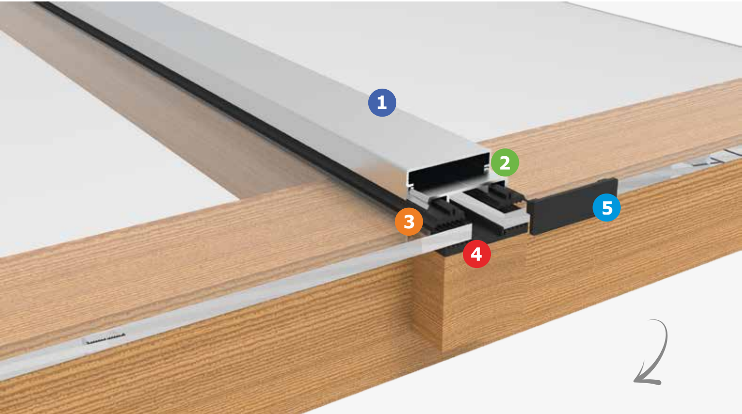
1. ALU-KLIPSDECKSCHIENE | 2. ALU-FLACHDECKSCHIENE | 3. DICHUNGSGUMMI | 4. AUFLEGEBAND | 5. XXXXXXXXXXXXXXXXXXXXXXXX
